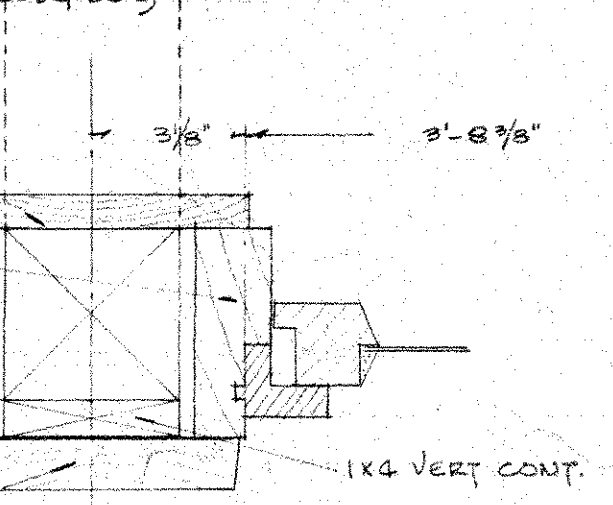
PLAN 48/16
