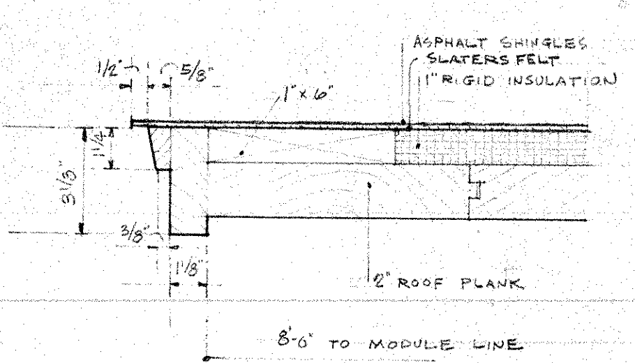
DETAIL 94 SCALE: 3" = 1'-0"
