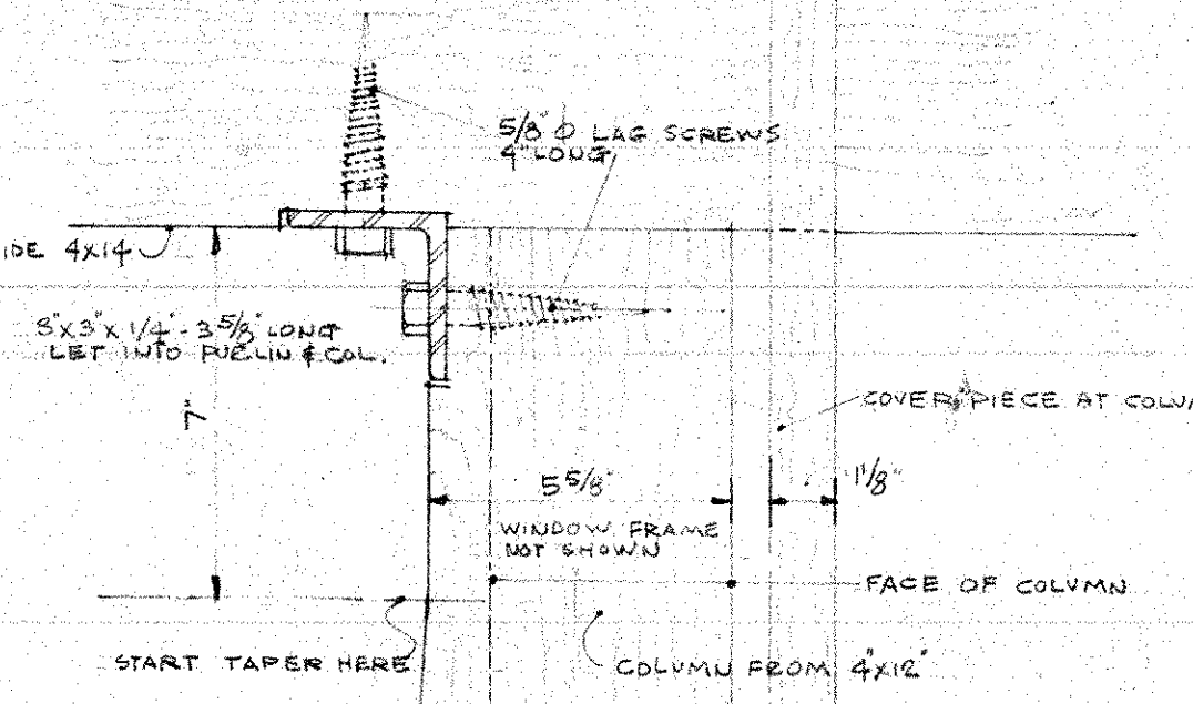
DETAIL 96 SCALE: 3" = 1'-0"
