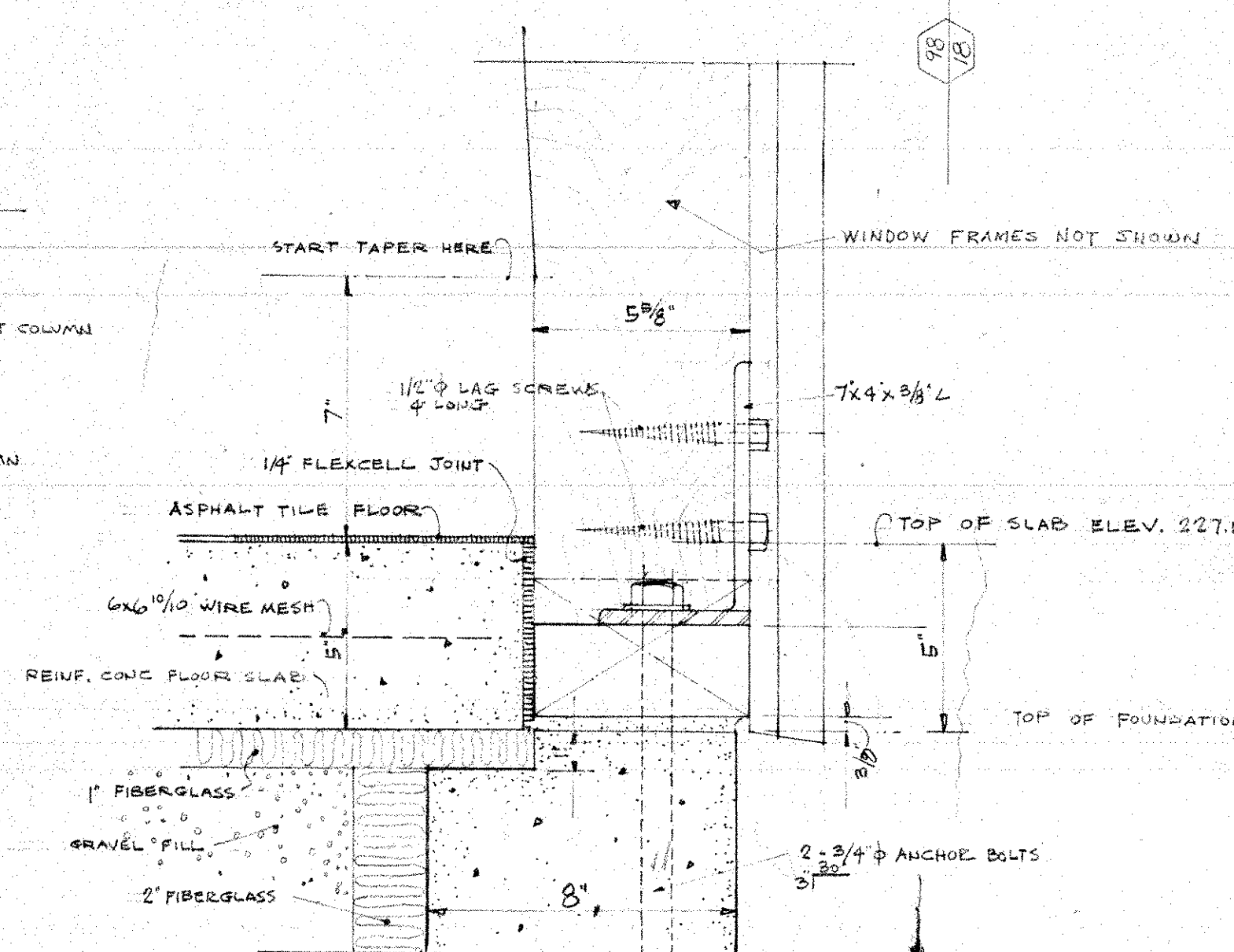
DETAIL 97 SCALE: 3" = 1'-0"
