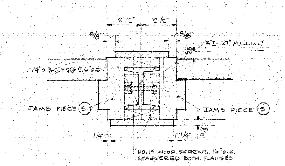
DETAIL 99 SCALE: 3" = 1'-0"
