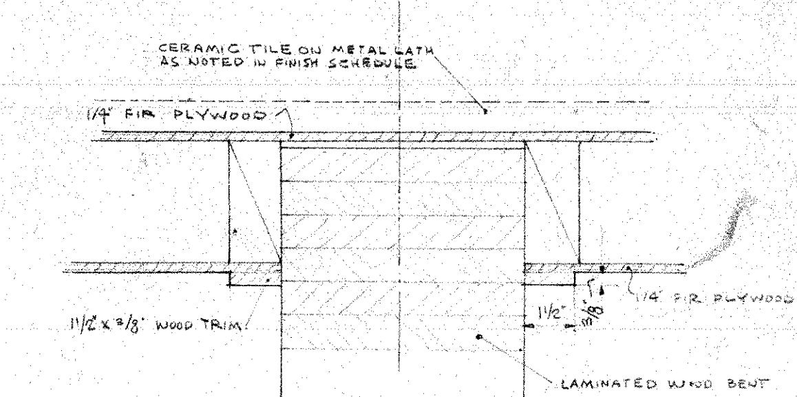
DETAIL 100 SCALE: 3" = 1'-0"
