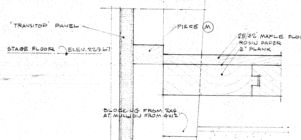
DETAIL 95 SCALE: 3" = 1'-0"
